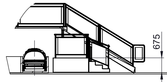
SEZIONE B-B SCALA 1 : 100
